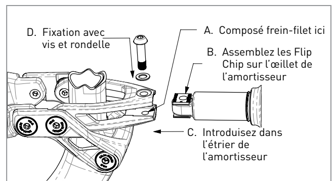
Figure 3 - Procédure d'assemblage
