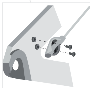
CAPTEUR DE VITESSE
