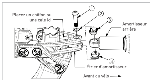
Figure 1 - Vue éclatée
